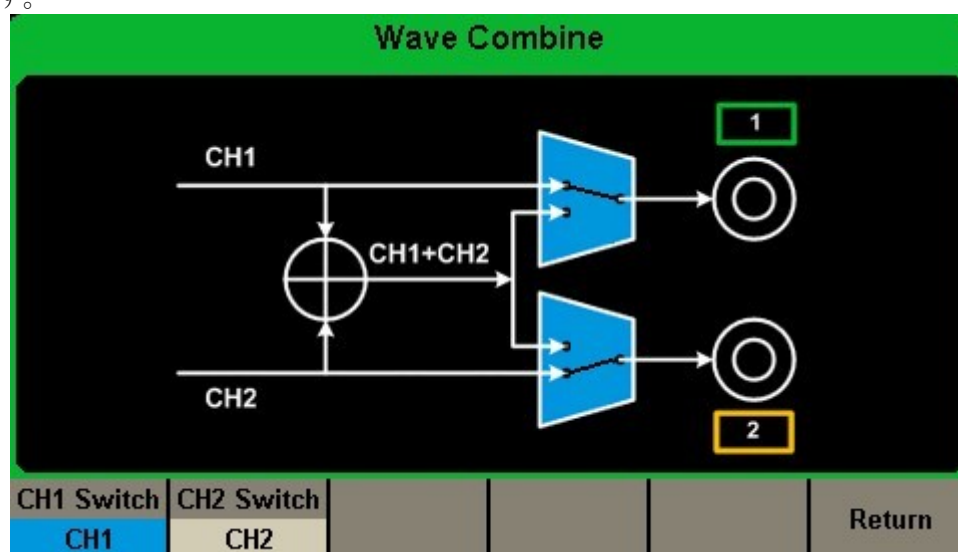
図 2-66 波形合成インタフェース
