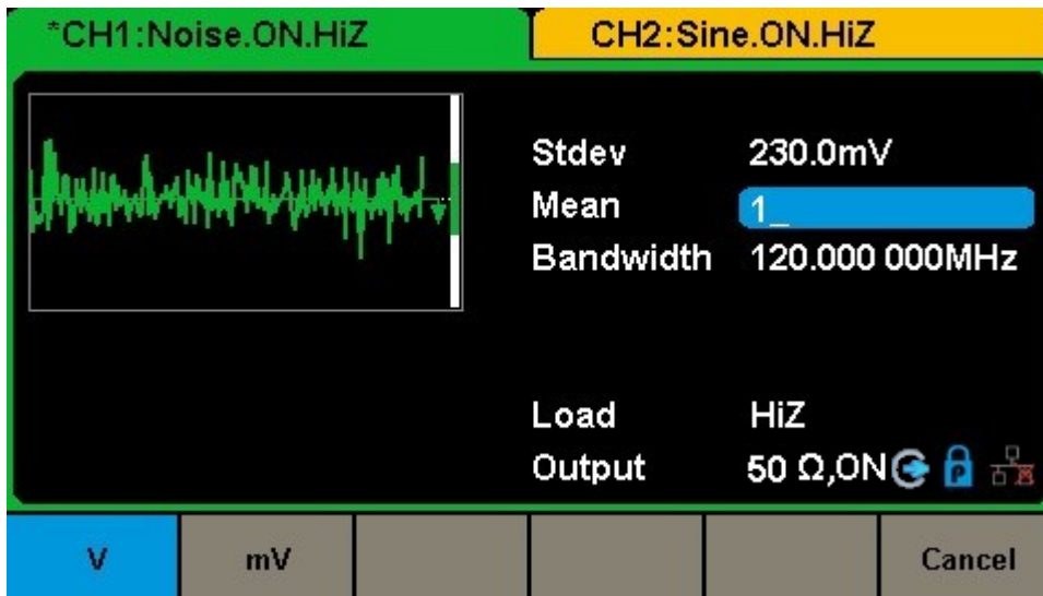
図 2-15 平均の設定
