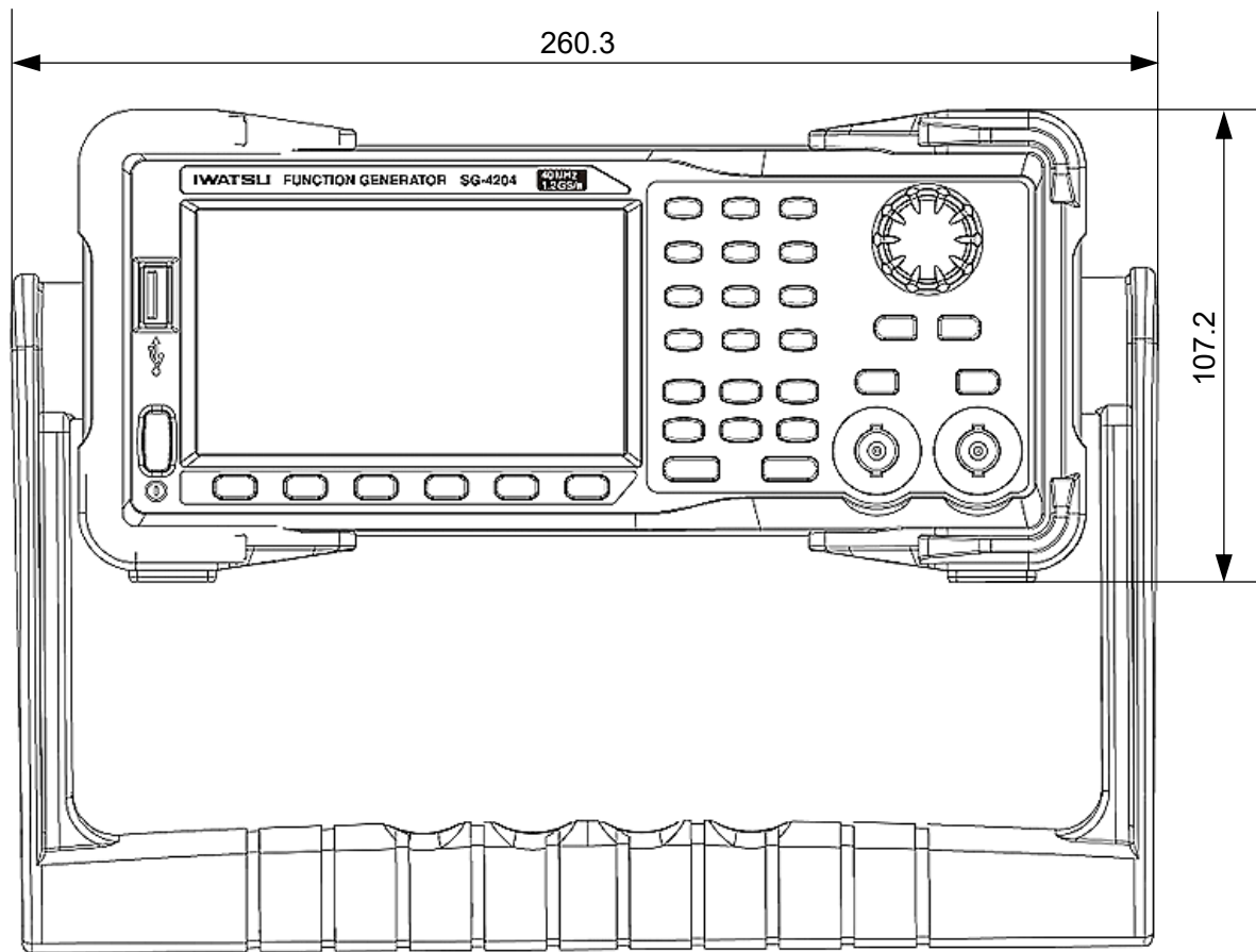
正面図
