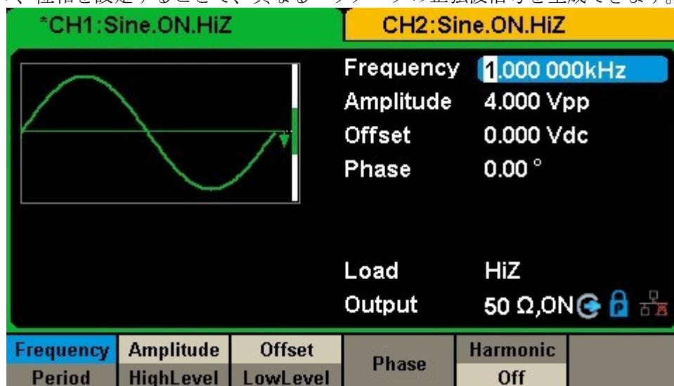
図 1-6 正弦波生成時のインターフェース
