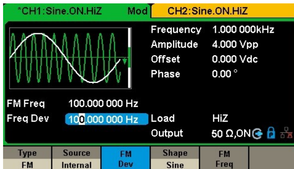
図 2-26 FM 設定インタフェース
