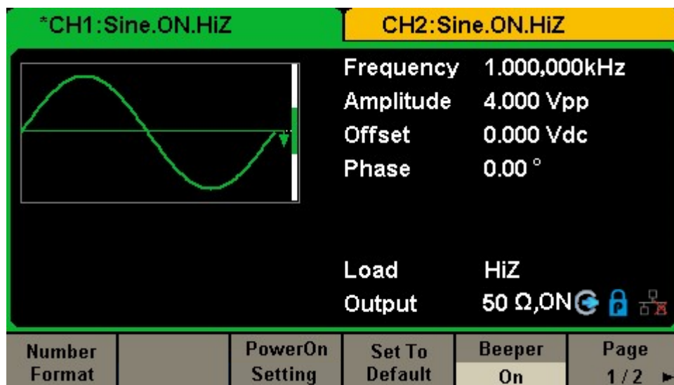
図 2-48 システム設定インタフェース(ページ 1/2)
