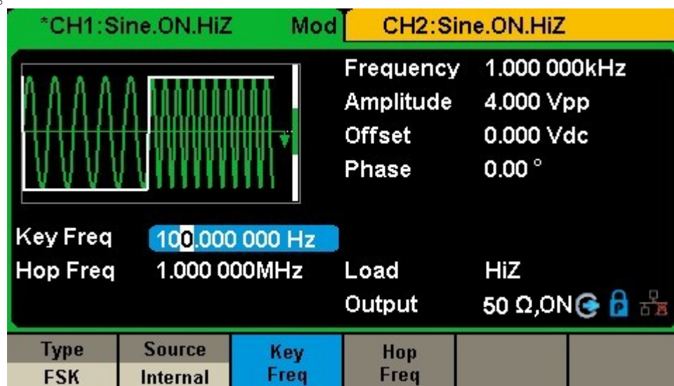
図 2-28 FSK 設定インターフェース
