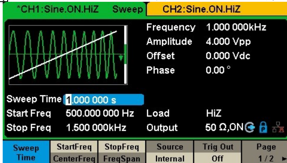
図 2-34 Sweep設定インタフェース (ページ 1/2)
