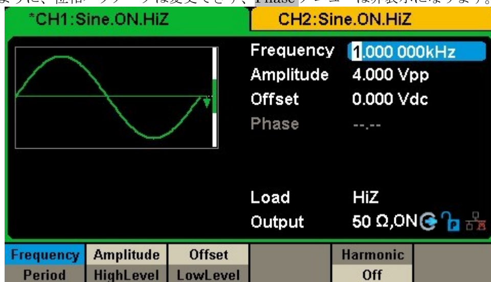
図 2-77 独立モード
