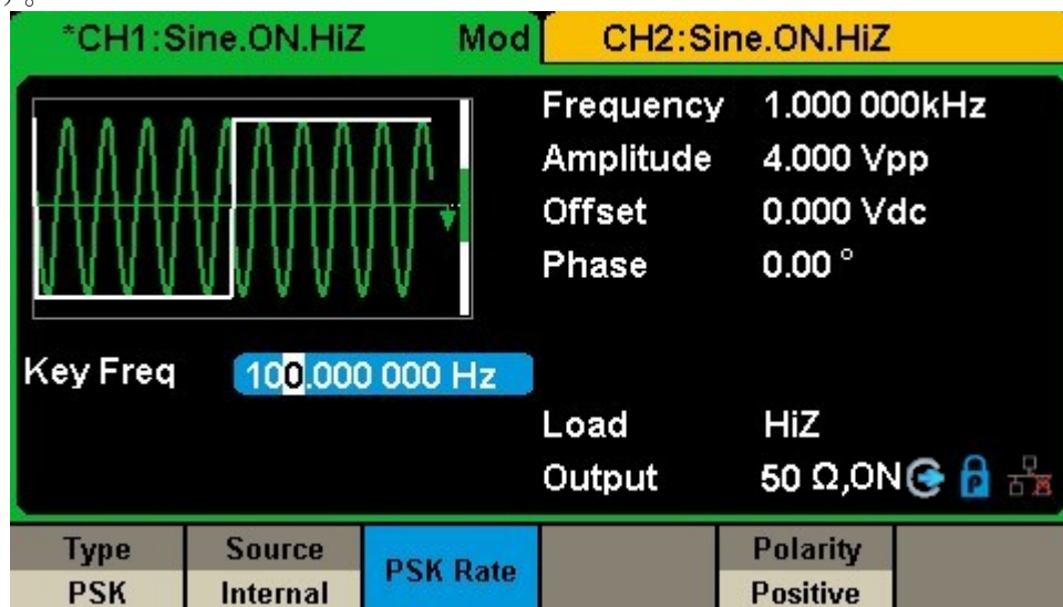
図 2-30 PSK 設定インターフェース
